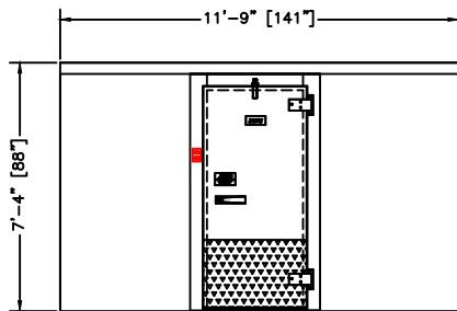
ELEVATION RIGHT HINGE
