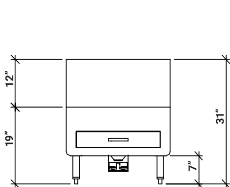
ELEVATION
