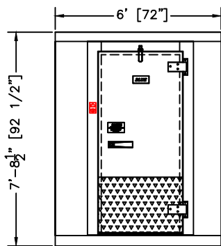
ELEVATION RIGHT HINGE
