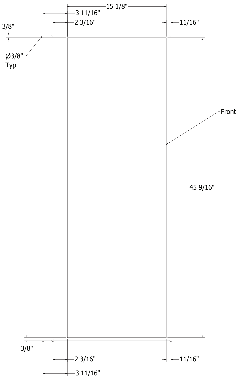
Cutout Template
