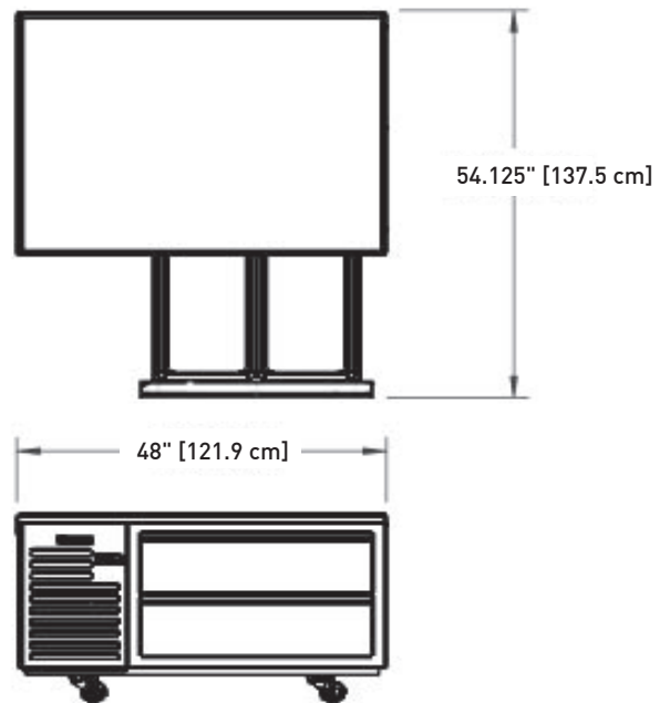
Elevation - TE048HT
