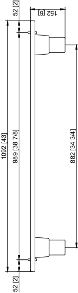
Seitenansicht mit Standard Füßen Side view with standard feet Vue de côté avec pieds standards
