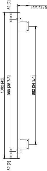
Seitenansicht mit niedrigen Füßen Side view with short feet Vue de côté avec pieds bas
