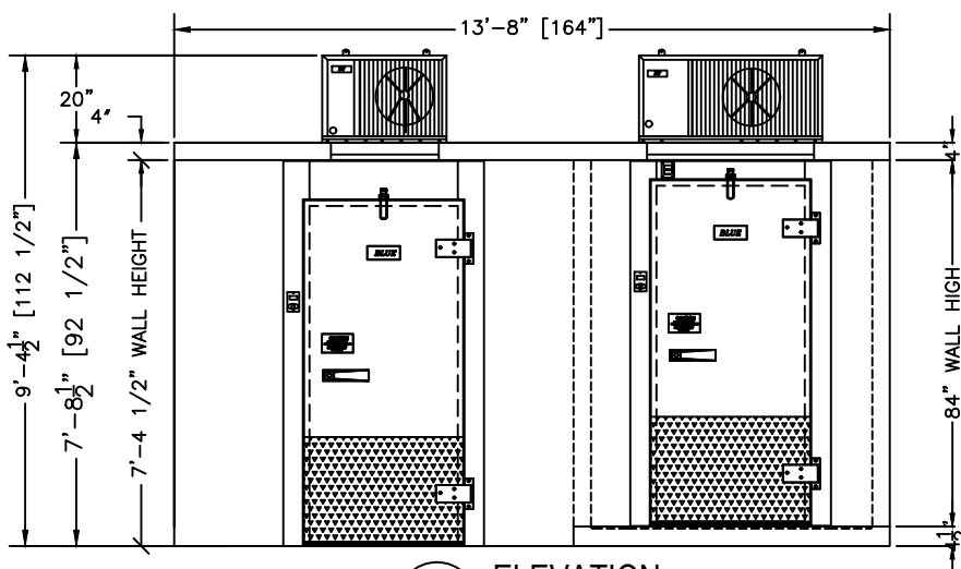
1 ELEVATION
