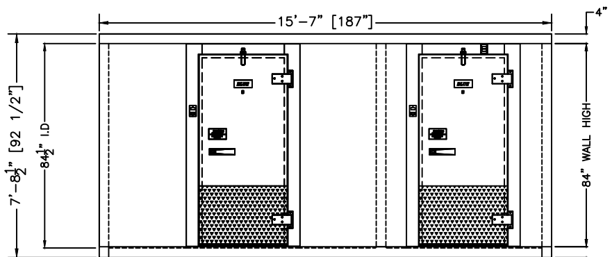
1 ELEVATION SCALE: 1/4"=1'-0"
