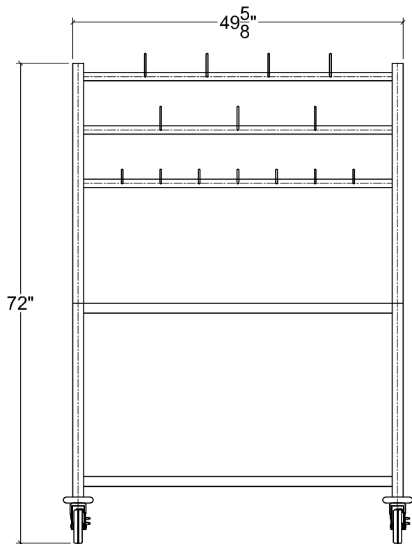
ELEVATION
