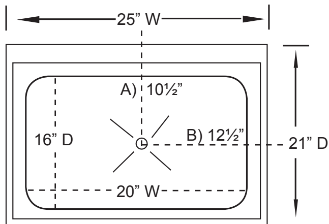
MS162012-CWP
