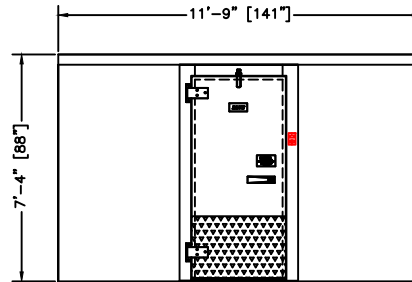
ELEVATION
