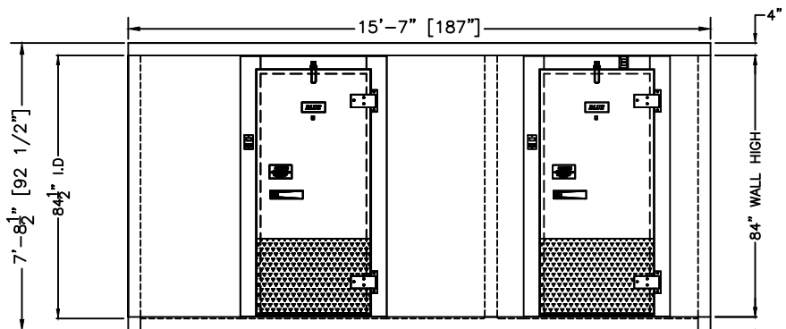
1 ELEVATION SCALE: 1/4"=1'-0"
