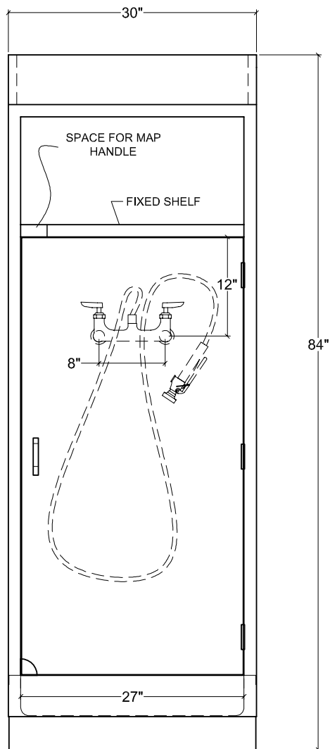
ELEVATION
