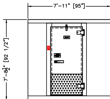
ELEVATION RIGHT HINGE
