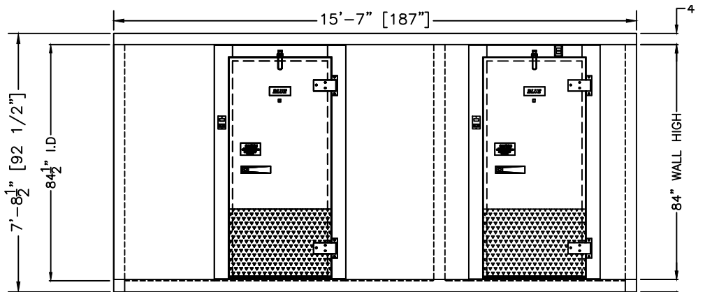
1 ELEVATION SCALE: 1/4"=1'-0"
