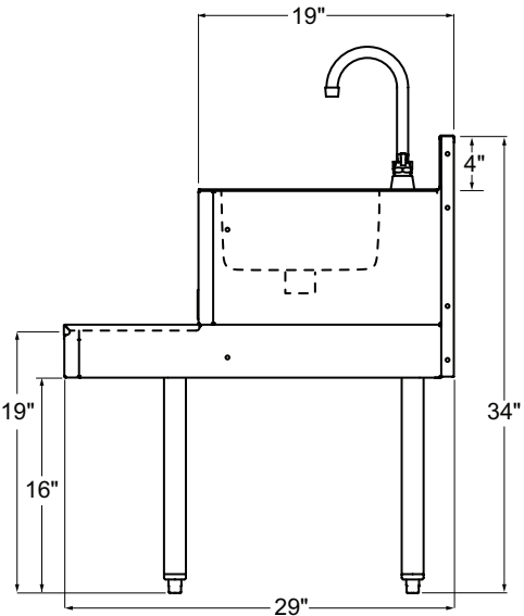
C-BSB-12, C-BSB-14, C-BSB-18 SIDE ELEVATION
