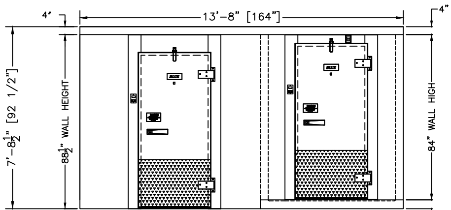
1 ELEVATION SCALE: 1/4"=1'-0"
