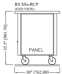
RS SSC-RCP-6 PANEL IN LIEU OF SHELF (ENCLOSED BASE)
