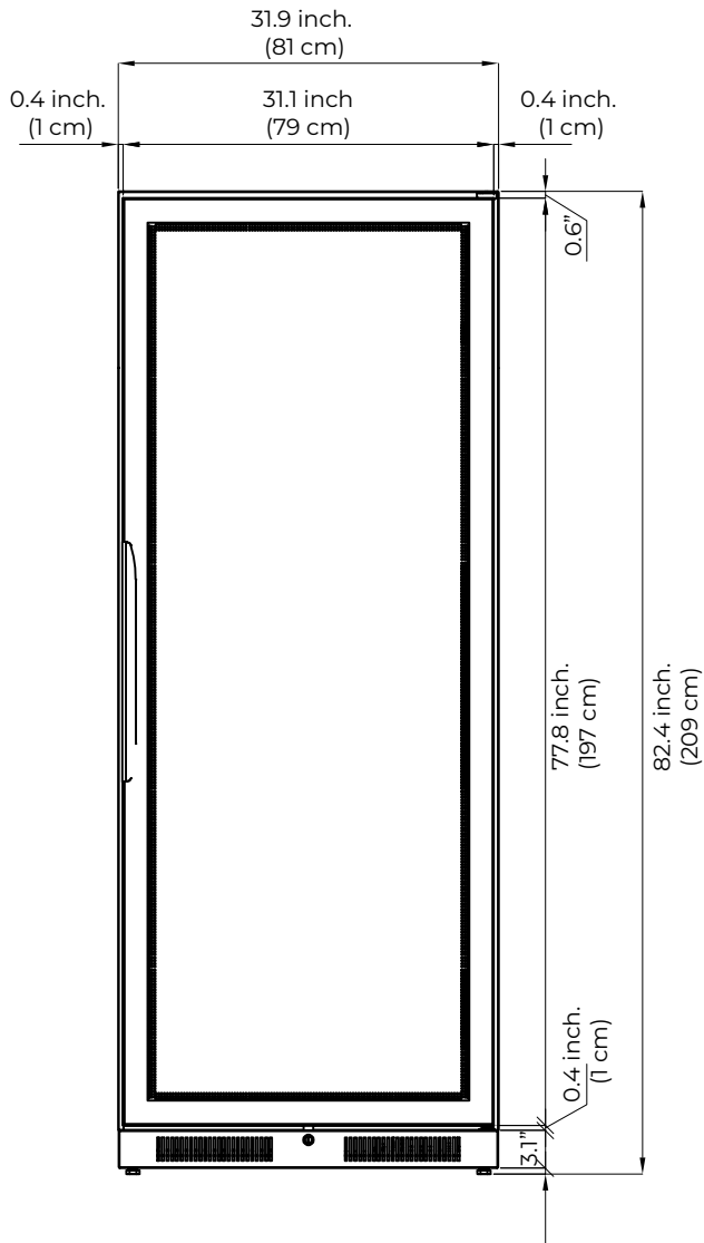
FRONTAL VIEW VUE AVANT
