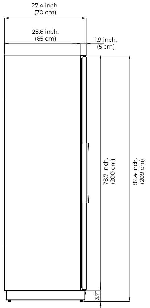
LEFT VIEW VUE DE CÔTÉ GAUCHE
