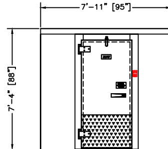
ELEVATION
