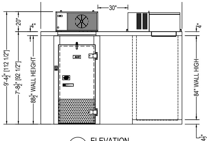
1 ELEVATION SCALE: 1/4"=1'-0"
