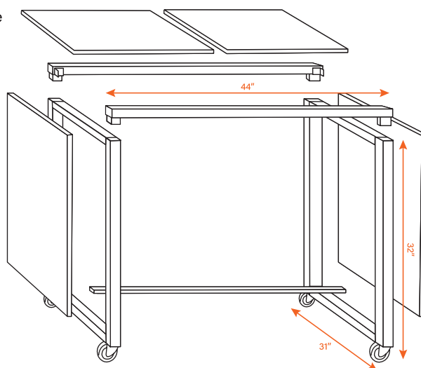
2 Tile Frame Z2010
