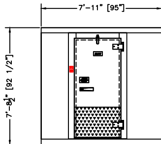
ELEVATION RIGHT HINGE
